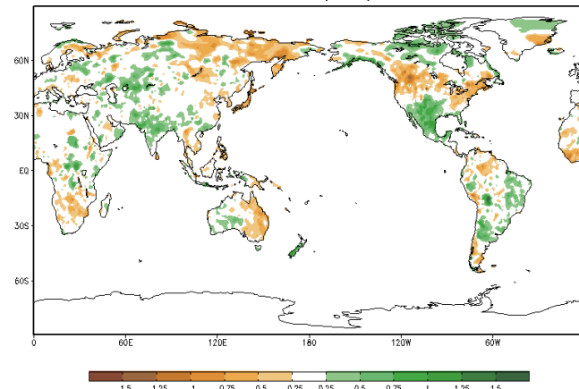
PDV DJF precip
