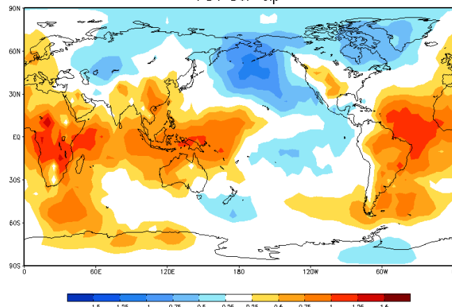
PDV DJF slp
