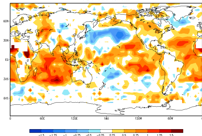
PDV JJA tanom
