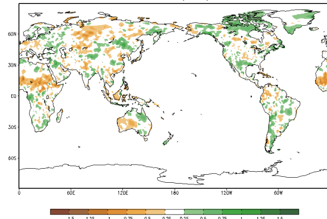
PDV JJA precip
