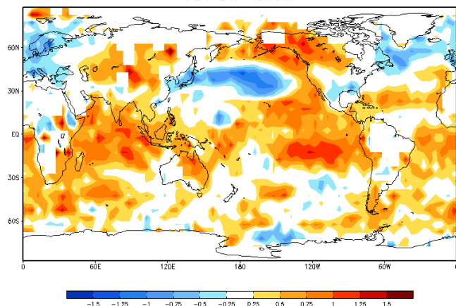
PDV DJF tanom
