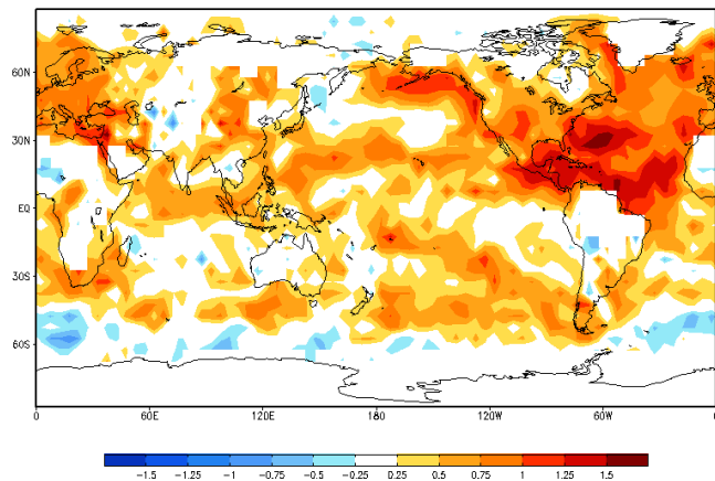
AMV JJA tanom
