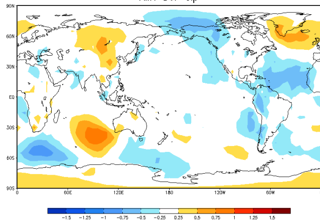
AMV DJF slp
