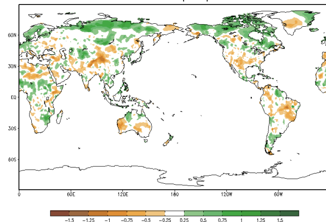
AMV JJA precip
