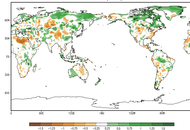
AMV DJF precip
