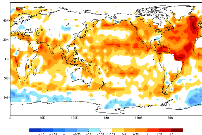
AMV DJF tanom
